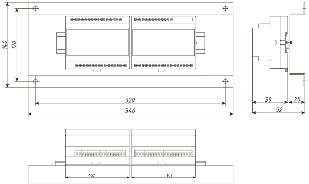
Периферийный блок
